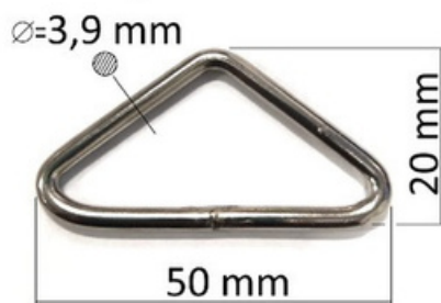
Anclaje triangular de camas elasticas
